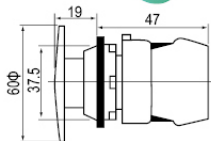
大头按钮 Big button
